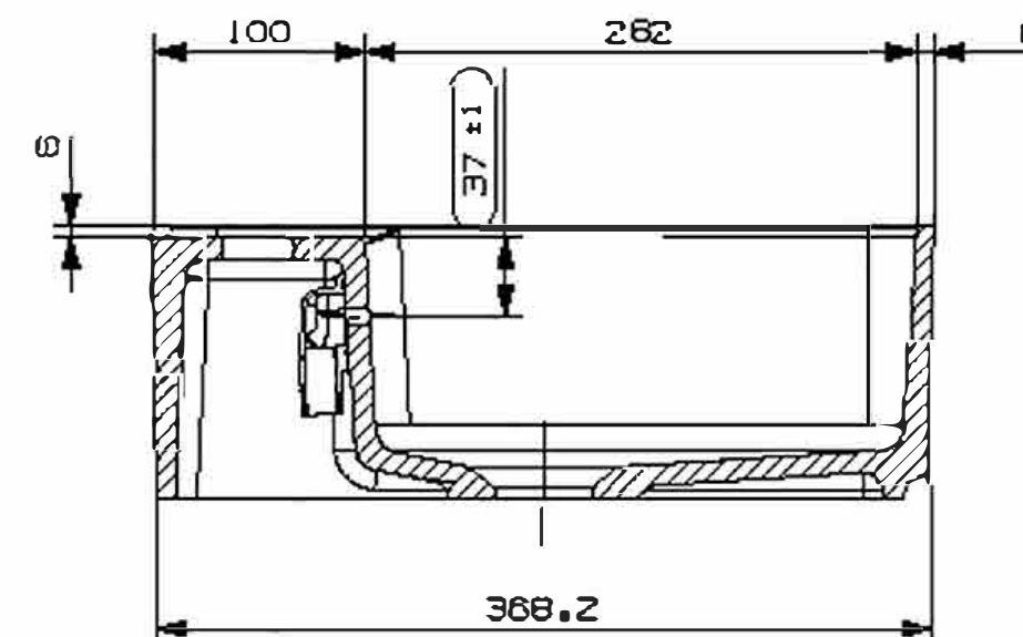
SECTION D-D SCALE 1:4
